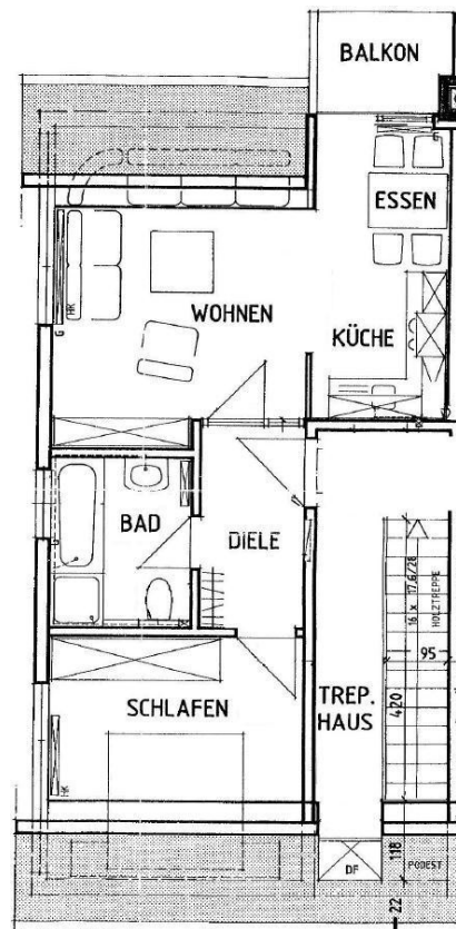
Grundriss
