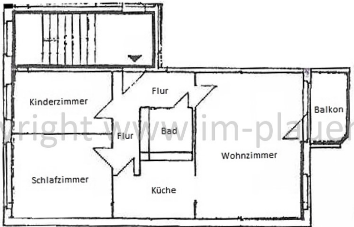
Grundriss
