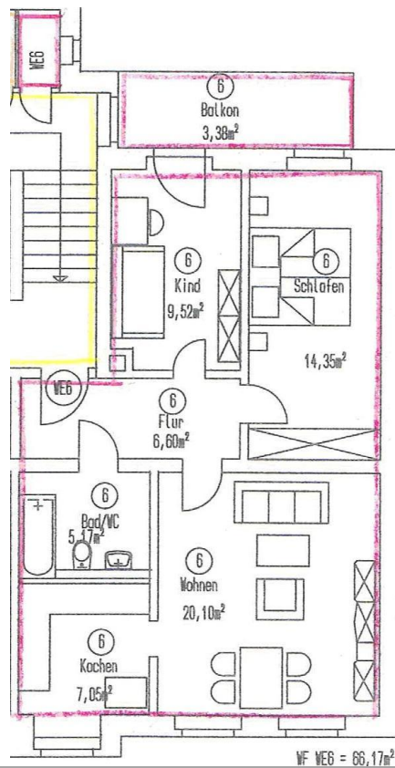
Wohnungsgrundriss
