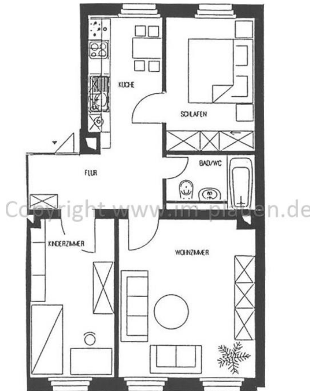
Grundriss
