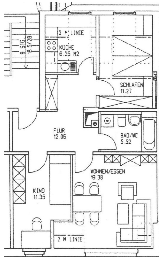
Grundriss - Hintere Gellertstraße 39 DG WHG 14 - K
