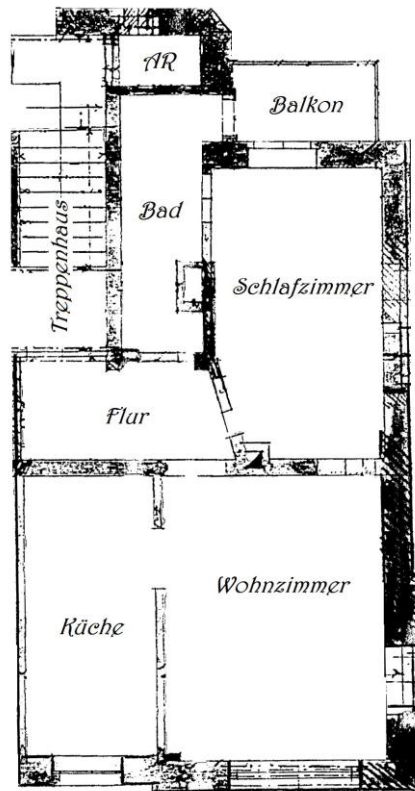
Grundriss
