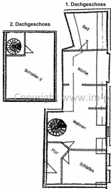
Grundriss
