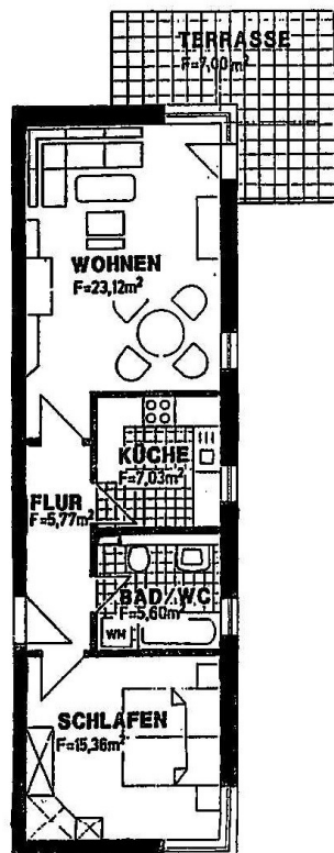
Grundriss
